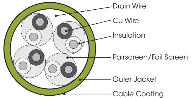
U/FTP
